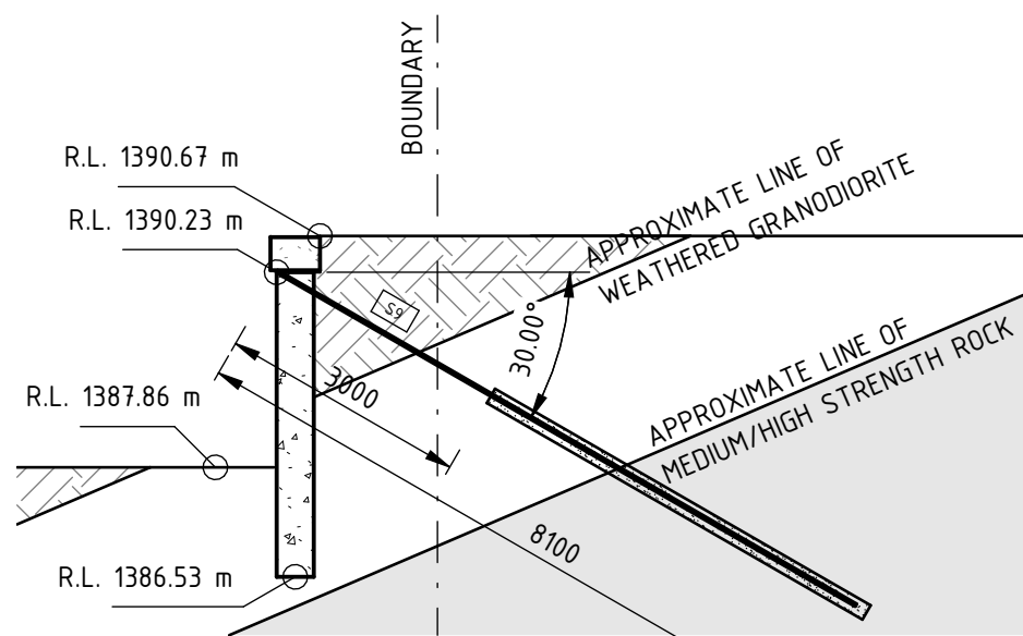
PILE S9
