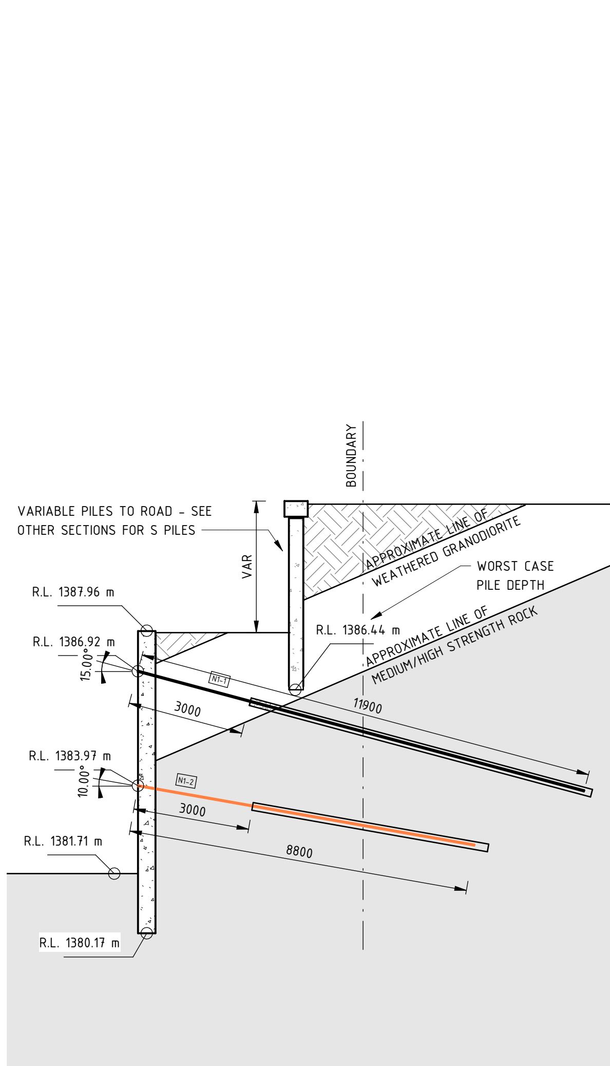
PILES N1
