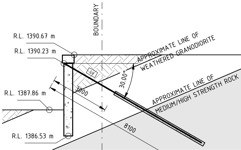
PILE S9
