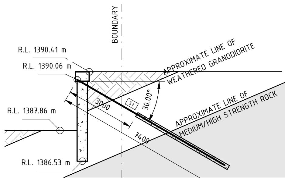
PILE S7
