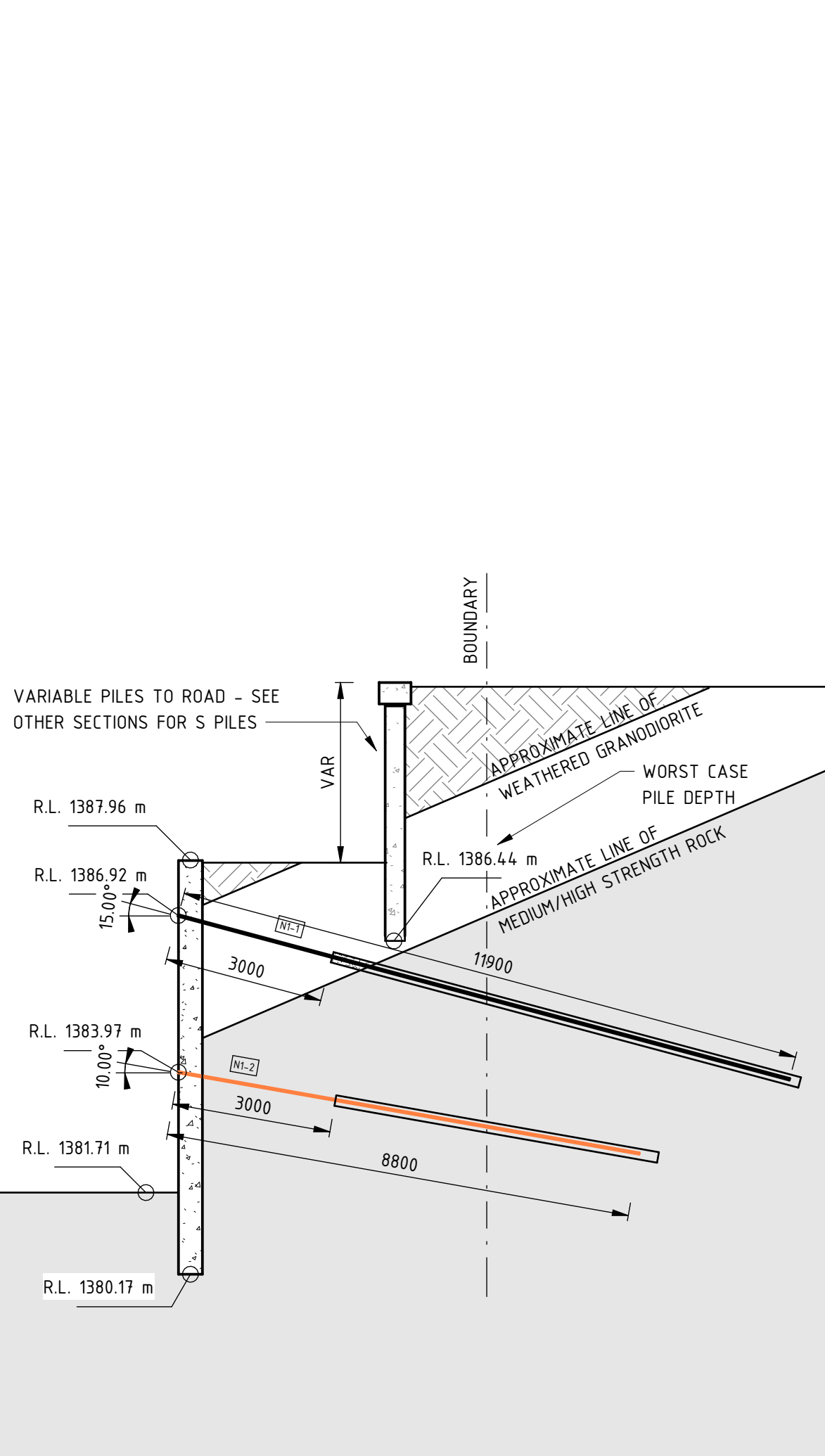
PILES N1
