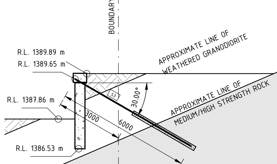
PILE S3
