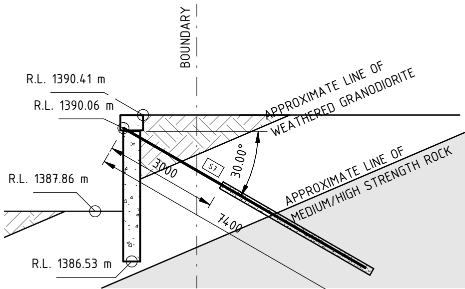
PILE S7
